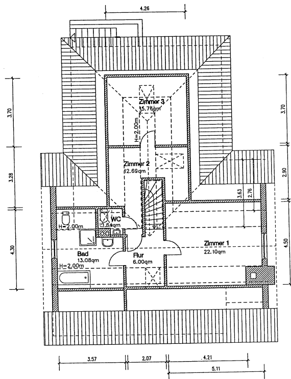
Dachgeschoss Nutzfläche ~71.27qm
